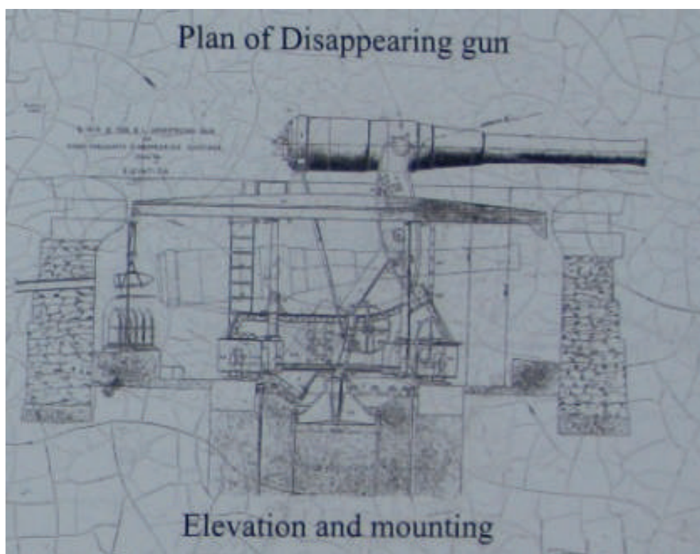
Рис. 4. Схема работы «исчезающей пушки» на Mount Victoria в Окленде.
